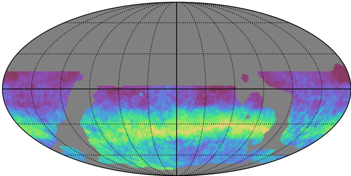
weather_cloudso6v3.4_10yrs WFD g band: AngleRms rotSkyPos
