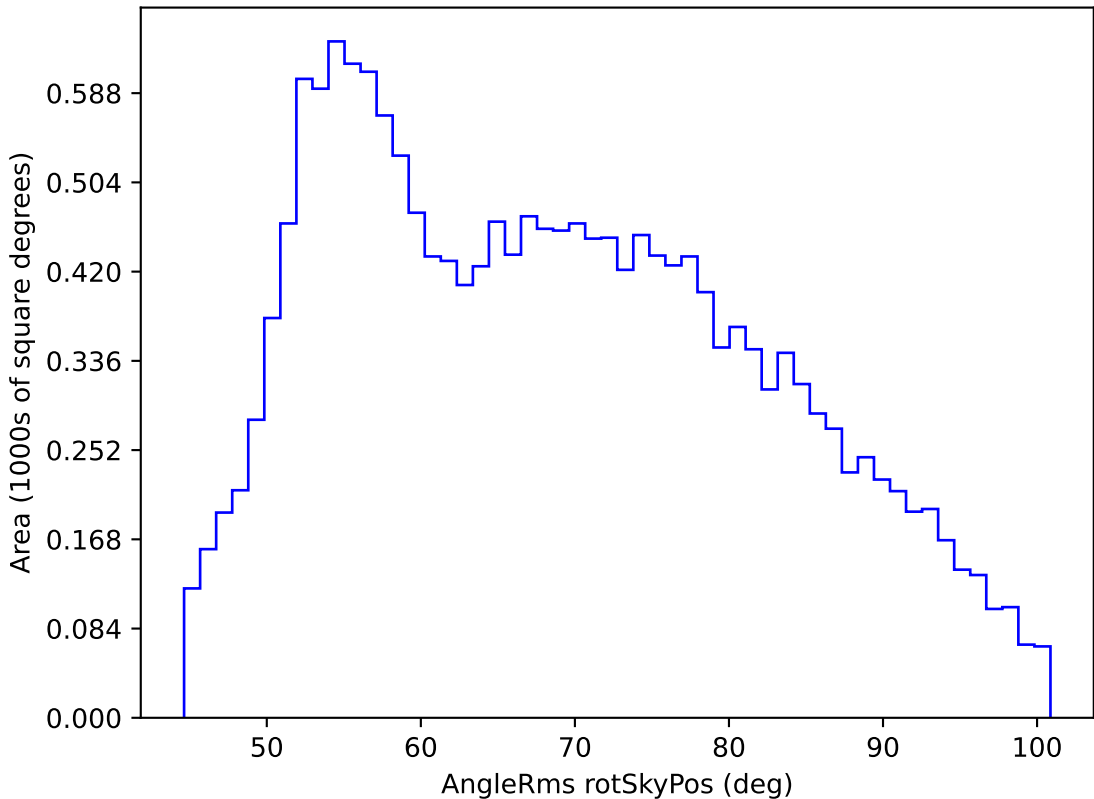
weather_cloudso6v3.4_10yrs WFD g band: AngleRms rotSkyPos
