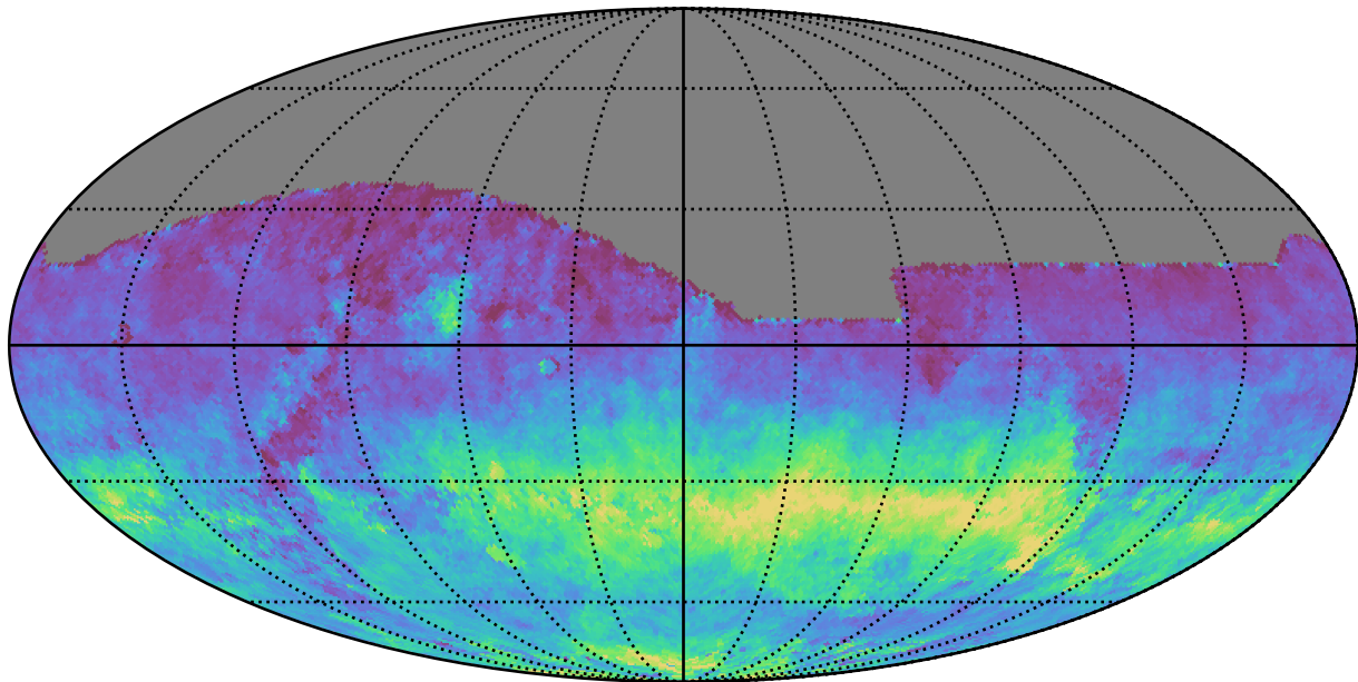
weather_cloudso6v3.4_10yrs All sky z band: AngleRms rotSkyPos
