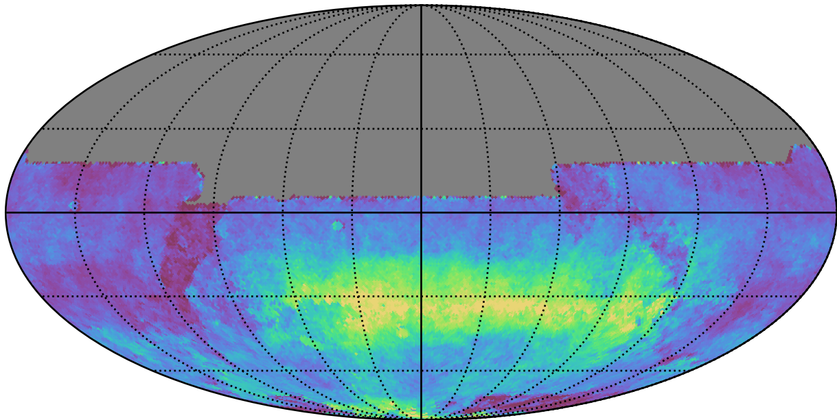
weather_cloudso6v3.4_10yrs All sky y band: AngleRms rotSkyPos
