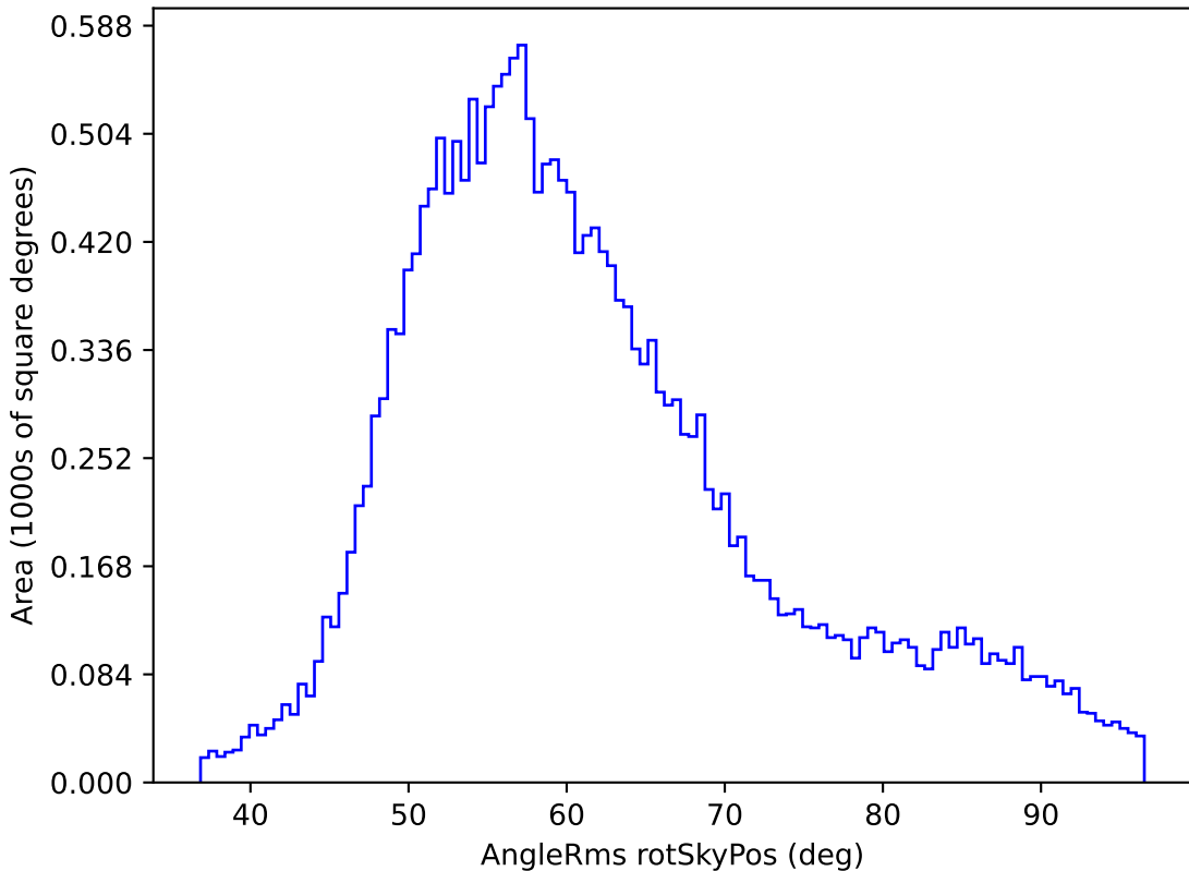
weather_cloudso6v3.4_10yrs All sky y band: AngleRms rotSkyPos
