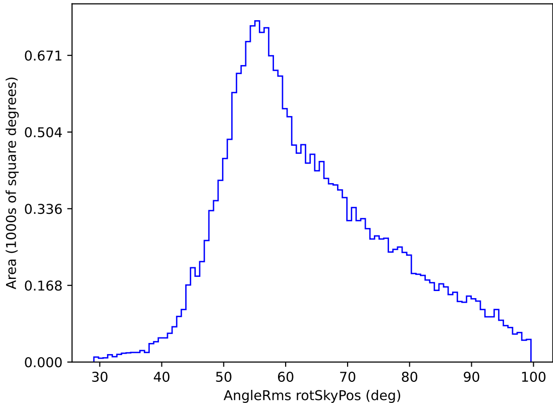
weather_cloudso6v3.4_10yrs All sky u band: AngleRms rotSkyPos
