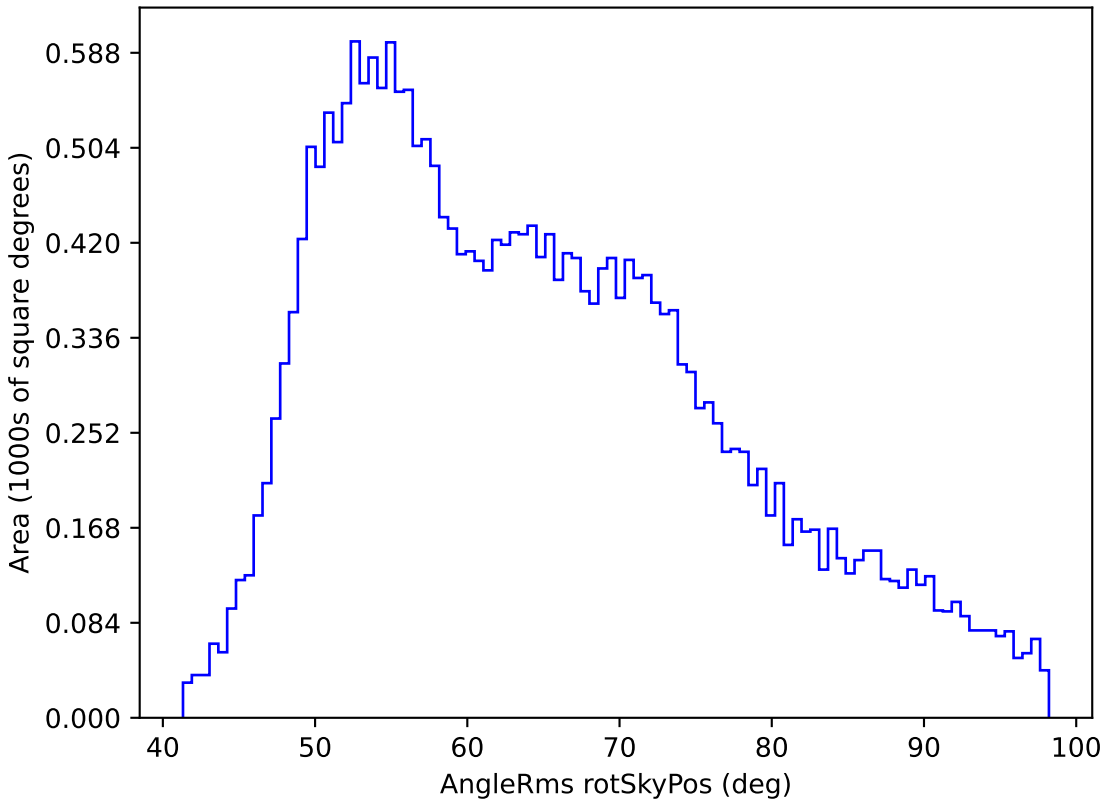
weather_cloudso6v3.4_10yrs All sky r band: AngleRms rotSkyPos
