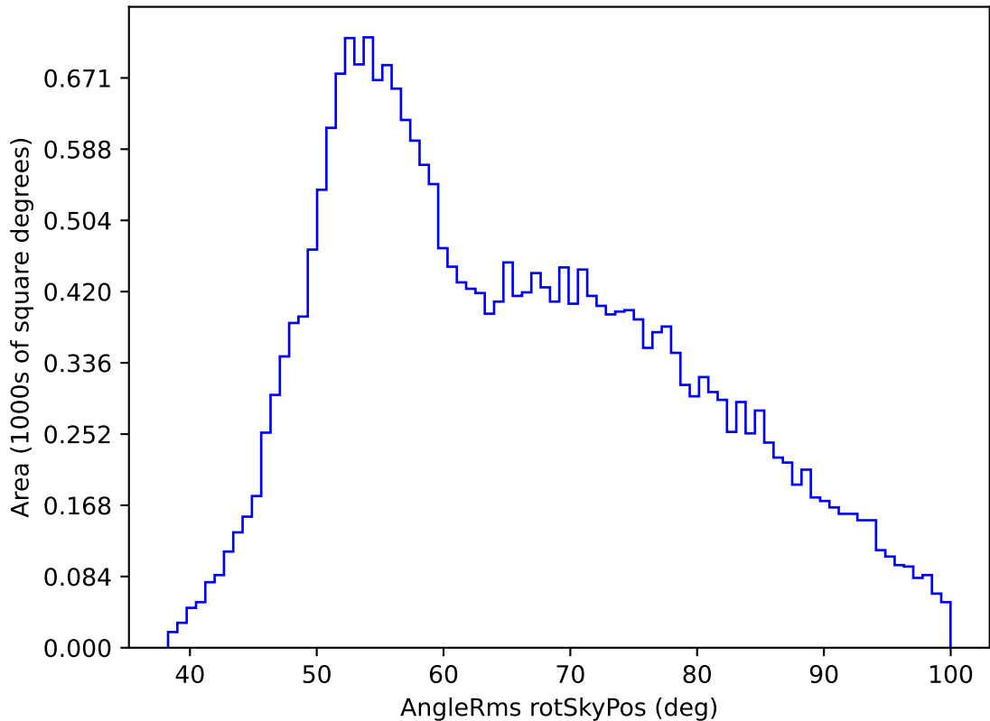
weather_cloudso6v3.4_10yrs All sky g band: AngleRms rotSkyPos
