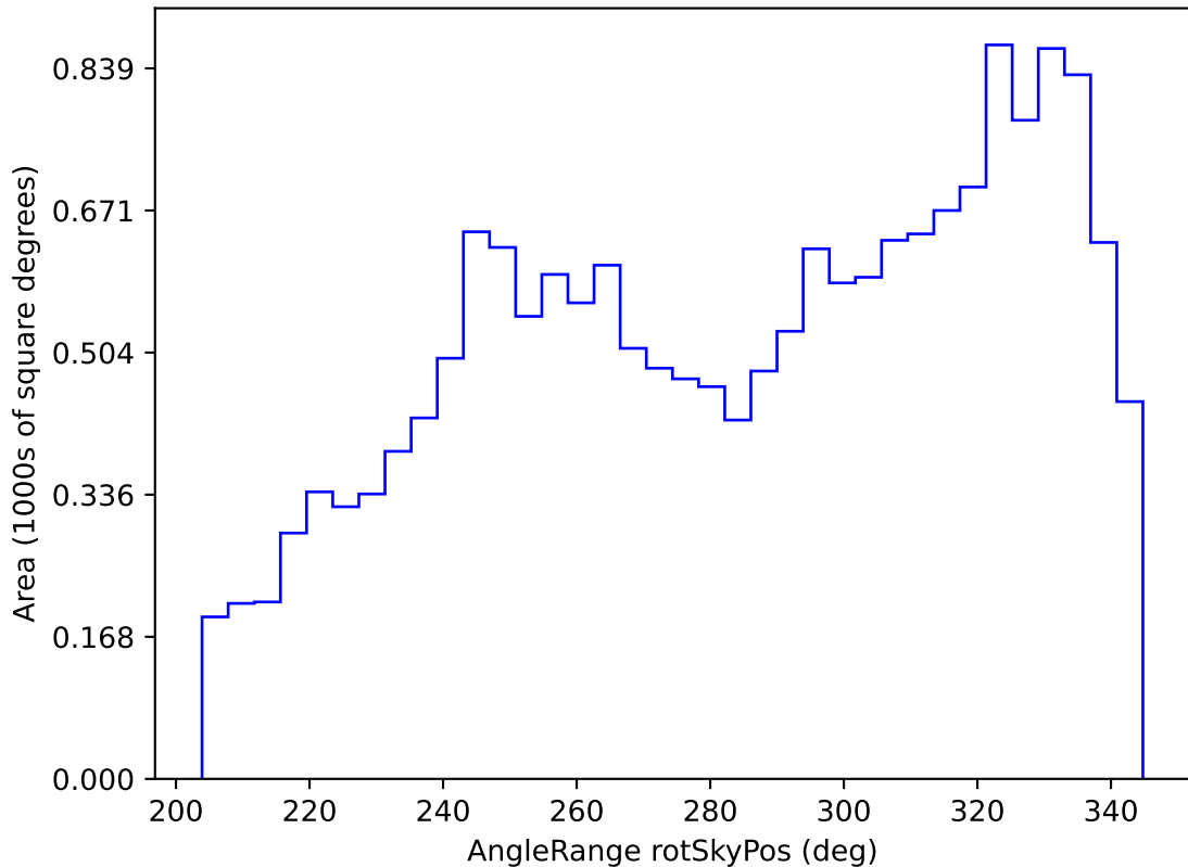
weather_cloudso6v3.4_10yrs WFD z band: AngleRange rotSkyPos
