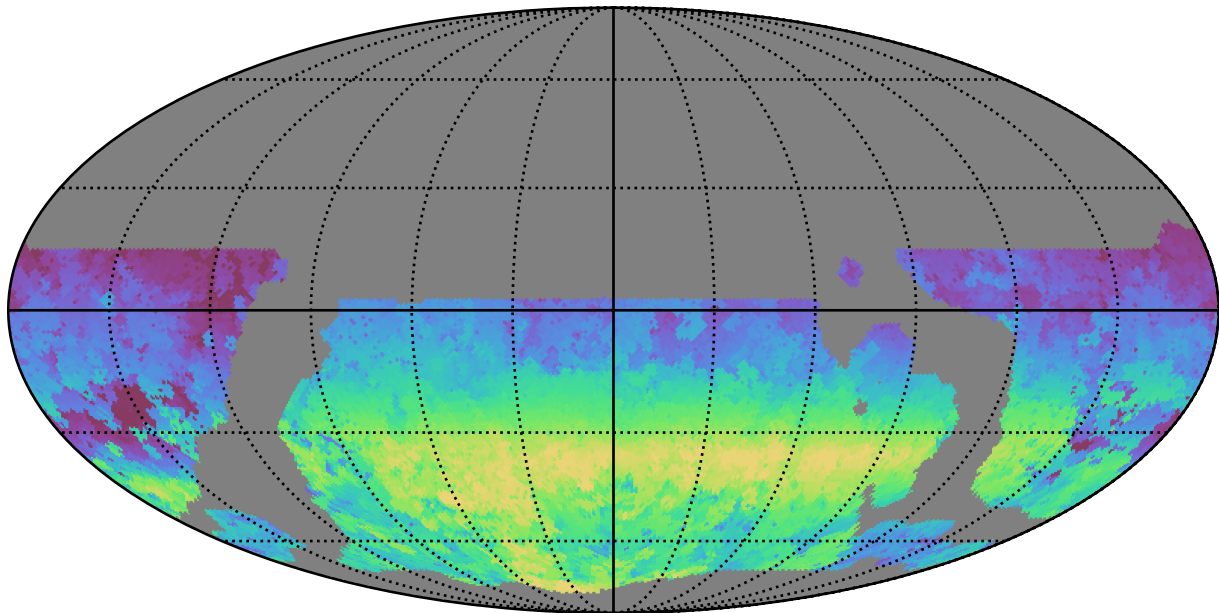
weather_cloudso6v3.4_10yrs WFD y band: AngleRange rotSkyPos
