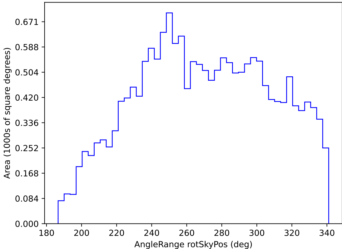
weather_cloudso6v3.4_10yrs WFD y band: AngleRange rotSkyPos
