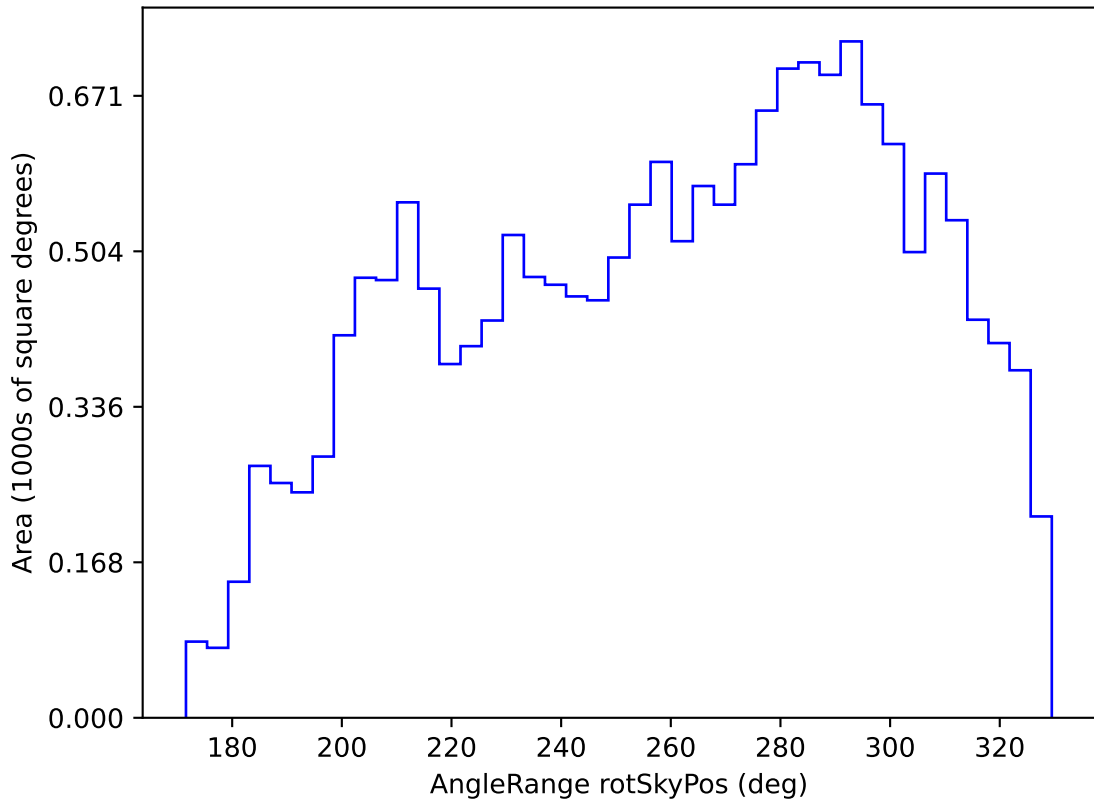
weather_cloudso6v3.4_10yrs WFD u band: AngleRange rotSkyPos
