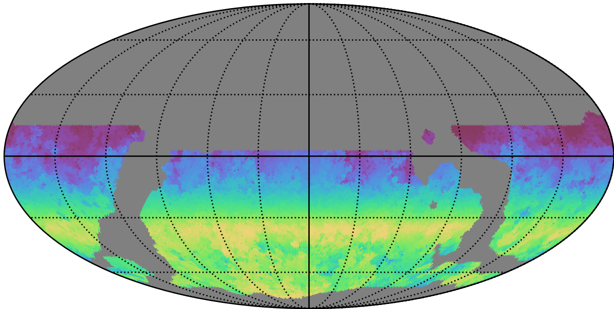
weather_cloudso6v3.4_10yrs WFD r band: AngleRange rotSkyPos
