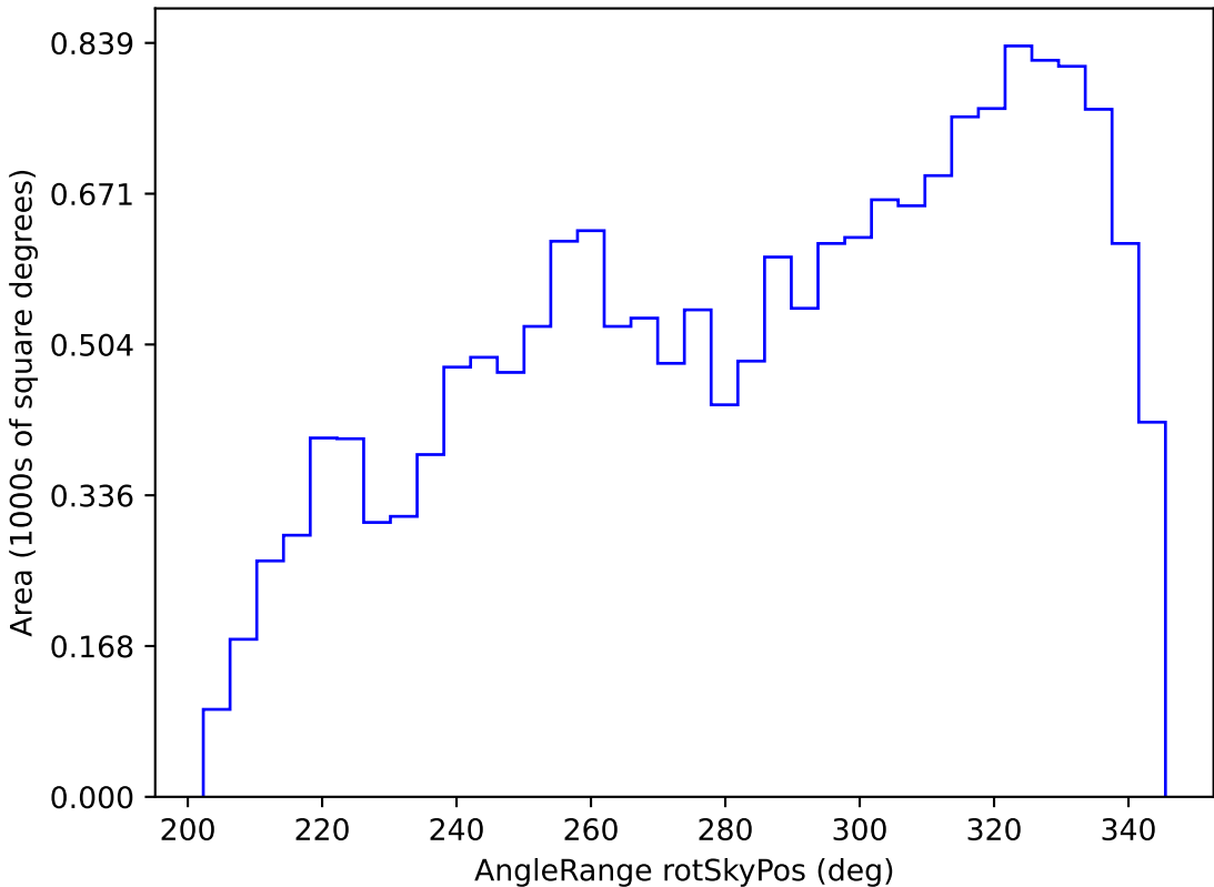
weather_cloudso6v3.4_10yrs WFD r band: AngleRange rotSkyPos
