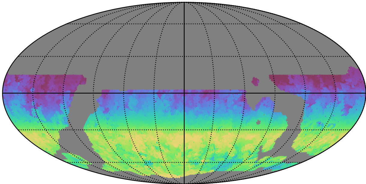
weather_cloudso6v3.4_10yrs WFD i band: AngleRange rotSkyPos
