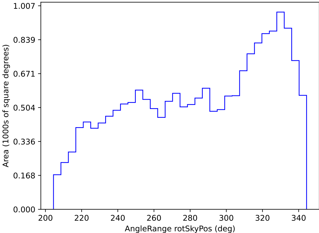
weather_cloudso6v3.4_10yrs WFD i band: AngleRange rotSkyPos
