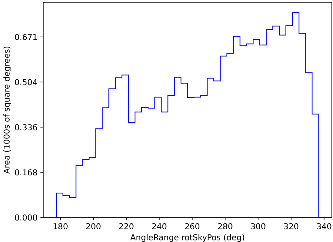
weather_cloudso6v3.4_10yrs WFD g band: AngleRange rotSkyPos
