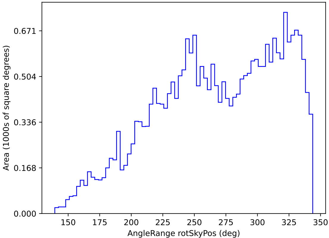
weather_cloudso6v3.4_10yrs All sky z band: AngleRange rotSkyPos
