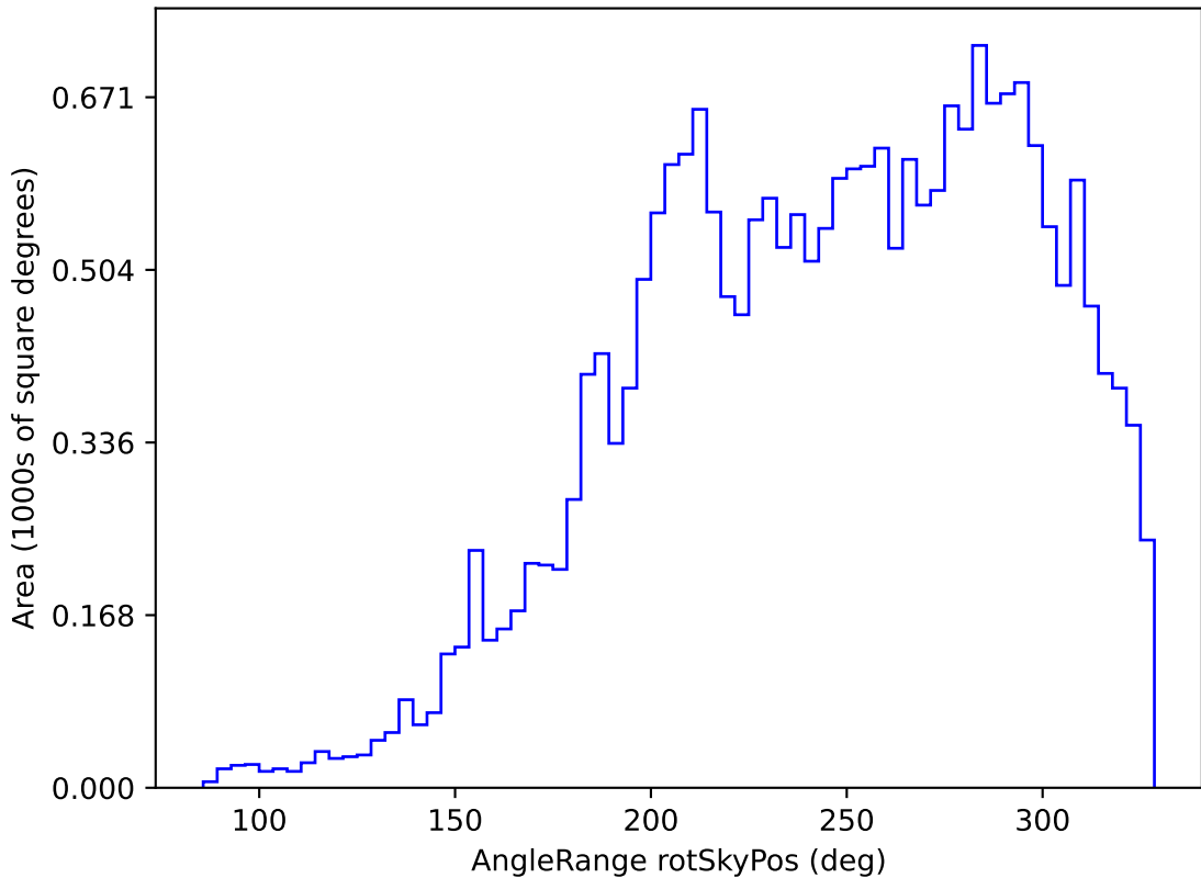
weather_cloudso6v3.4_10yrs All sky u band: AngleRange rotSkyPos
