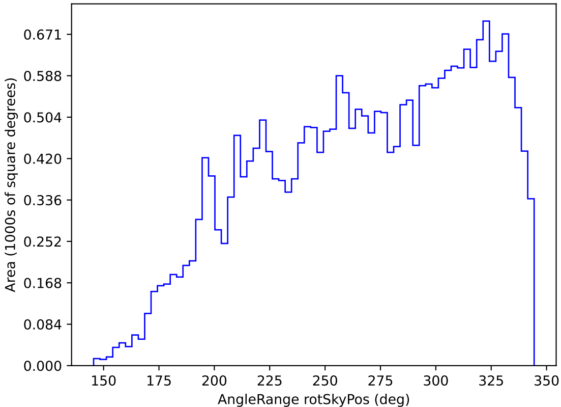
weather_cloudso6v3.4_10yrs All sky r band: AngleRange rotSkyPos
