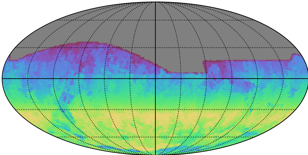
weather_cloudso6v3.4_10yrs All sky i band: AngleRange rotSkyPos
