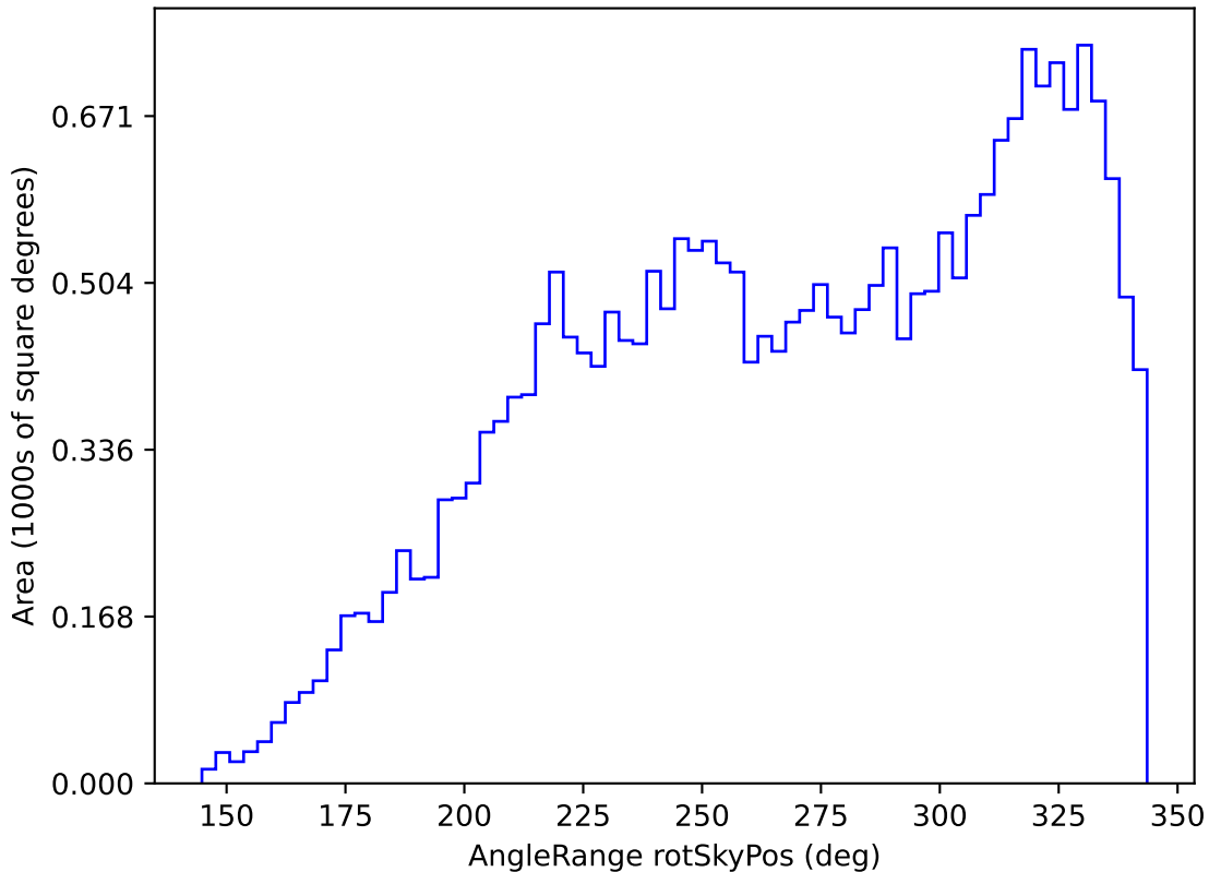
weather_cloudso6v3.4_10yrs All sky i band: AngleRange rotSkyPos
