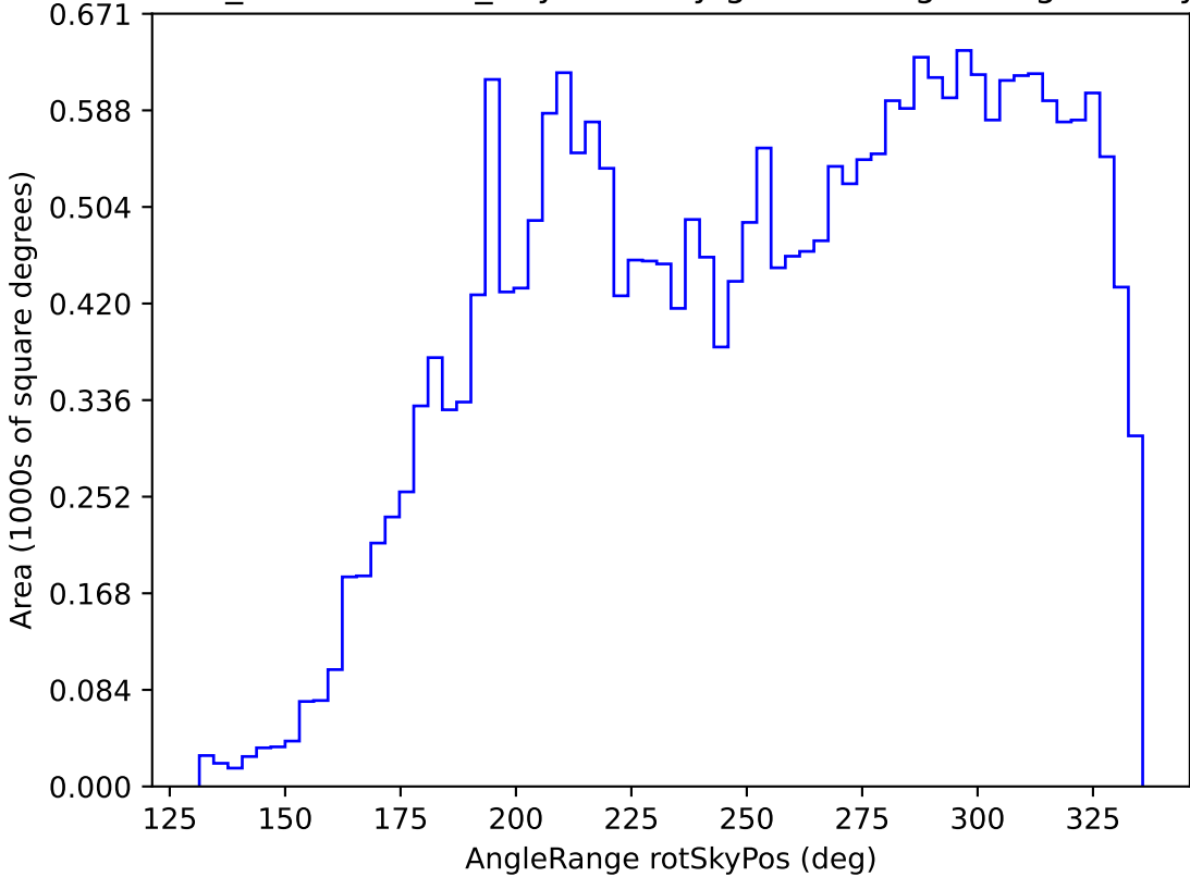
weather_cloudso6v3.4_10yrs All sky g band: AngleRange rotSkyPos
