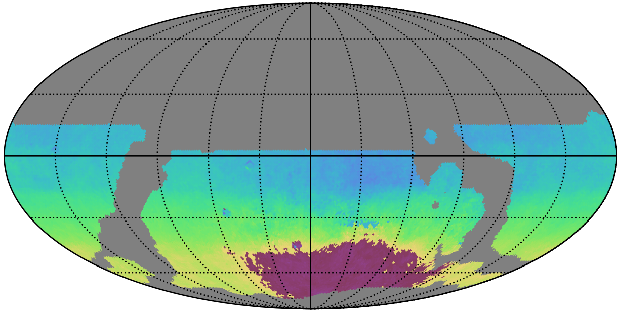
weather_cloudso6v3.4_10yrs WFD y band: AngleMean rotSkyPos
