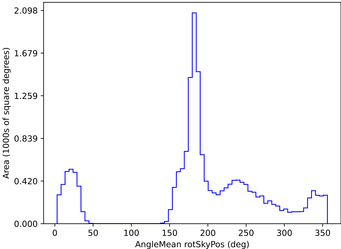
weather_cloudso6v3.4_10yrs WFD r band: AngleMean rotSkyPos
