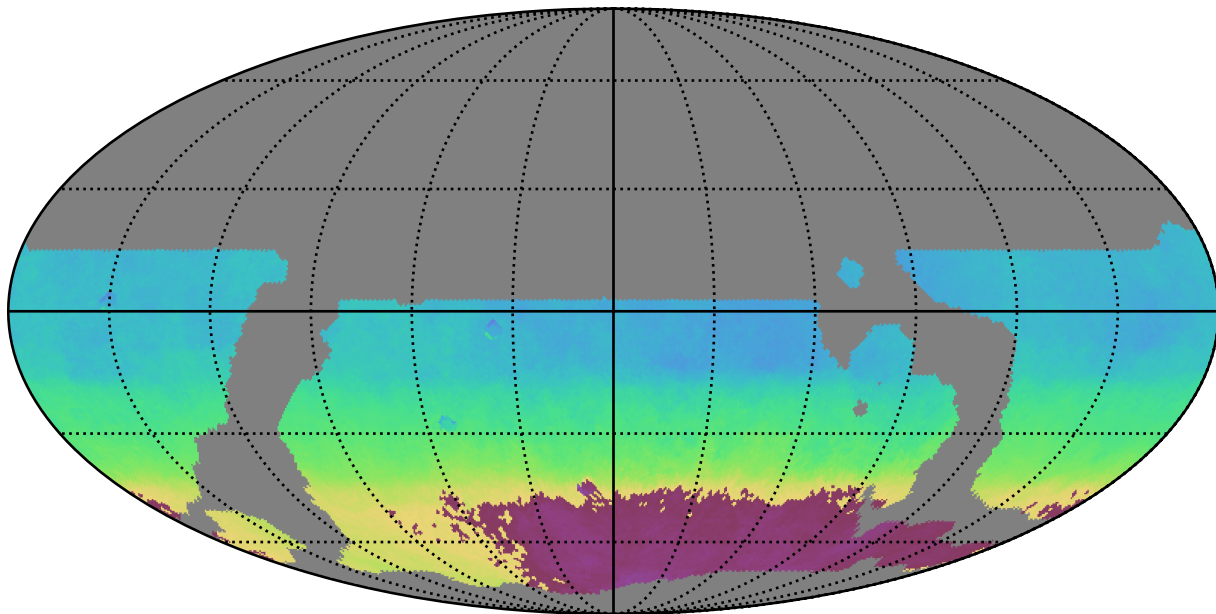
weather_cloudso6v3.4_10yrs WFD i band: AngleMean rotSkyPos
