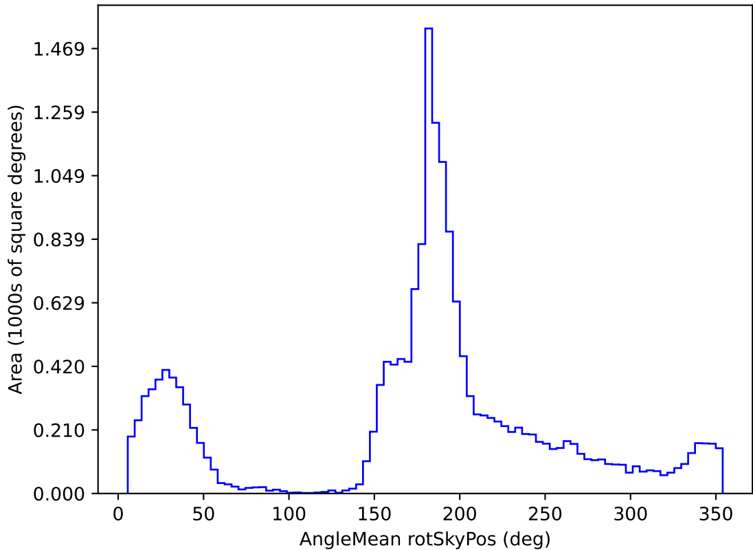
weather_cloudso6v3.4_10yrs WFD g band: AngleMean rotSkyPos
