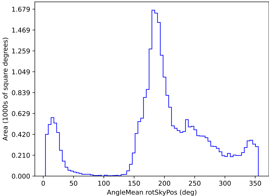
weather_cloudso6v3.4_10yrs All sky z band: AngleMean rotSkyPos
