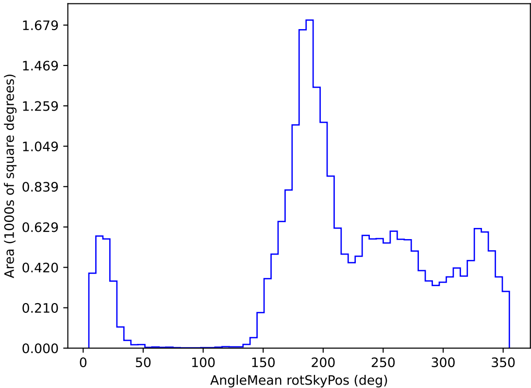
weather_cloudso6v3.4_10yrs All sky y band: AngleMean rotSkyPos
