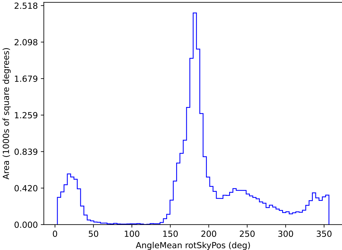
weather_cloudso6v3.4_10yrs All sky r band: AngleMean rotSkyPos
