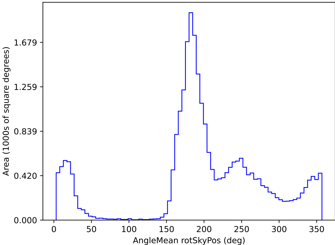
weather_cloudso6v3.4_10yrs All sky i band: AngleMean rotSkyPos
