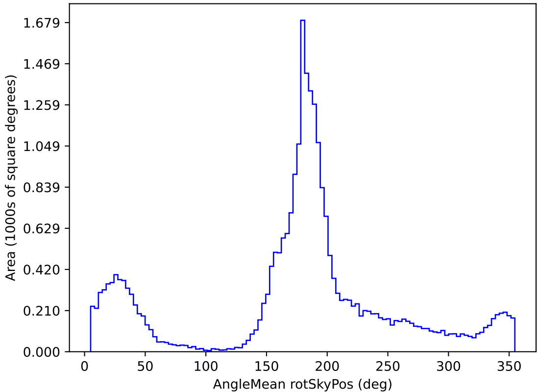
weather_cloudso6v3.4_10yrs All sky g band: AngleMean rotSkyPos
