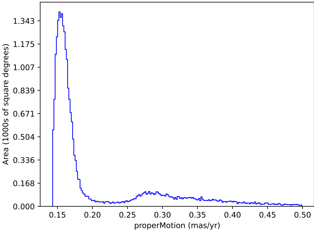
weather_cloudso6v3.4_10yrs : properMotion
