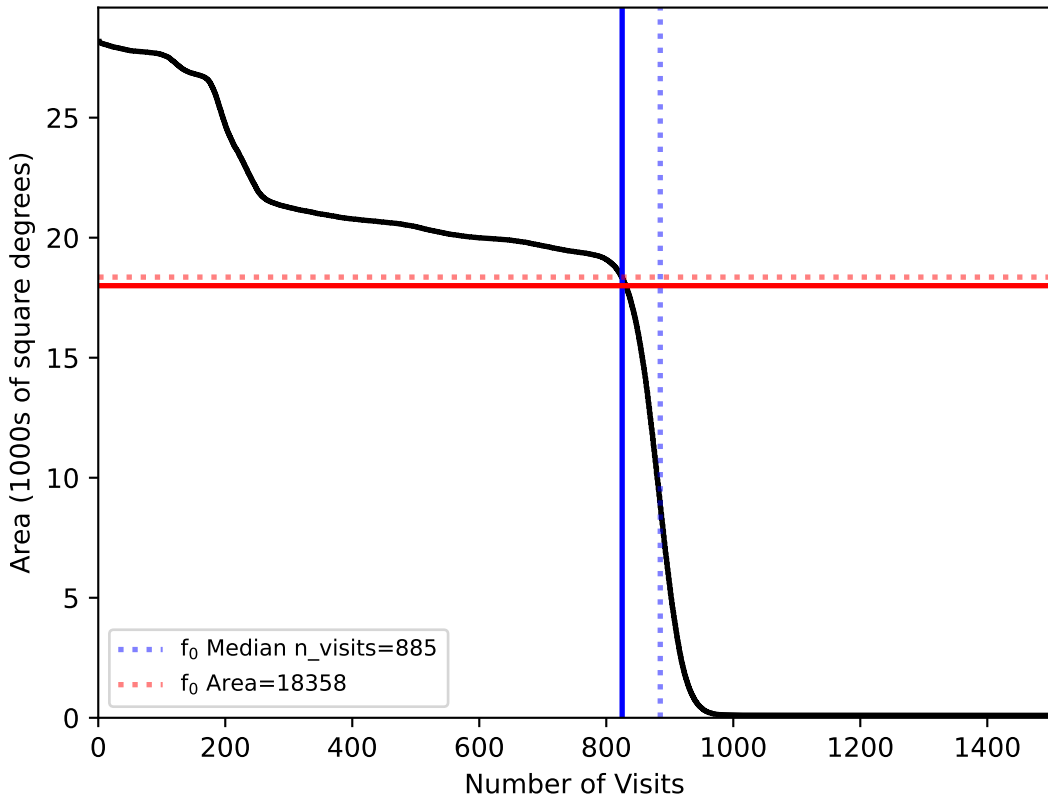
weather_cloudso6v3.4_10yrs : f0
