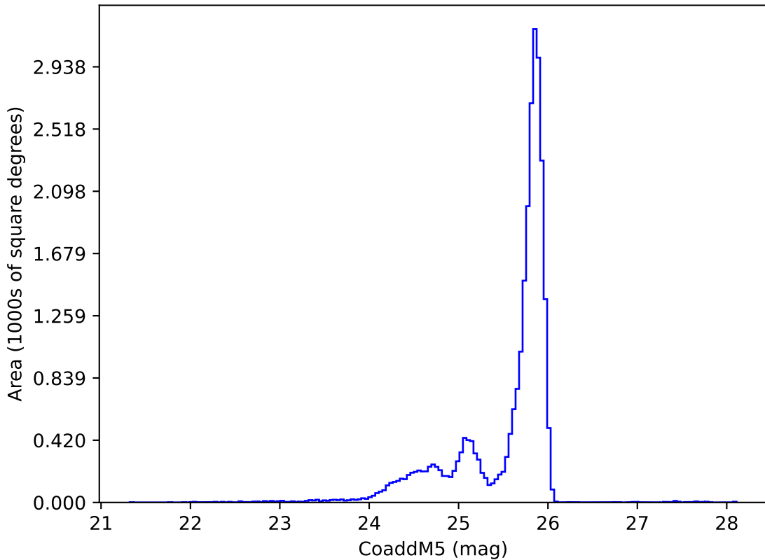
weather_cloudso6v3.4_10yrs z: CoaddM5
