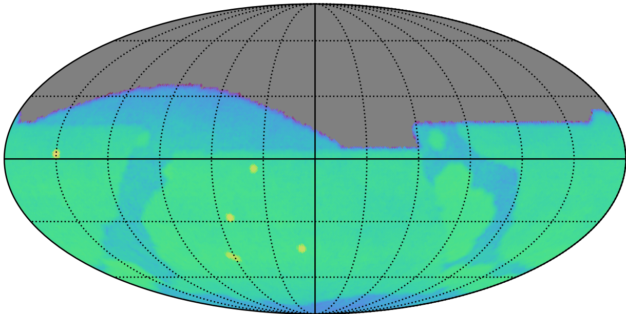
weather_cloudso6v3.4_10yrs g: CoaddM5
