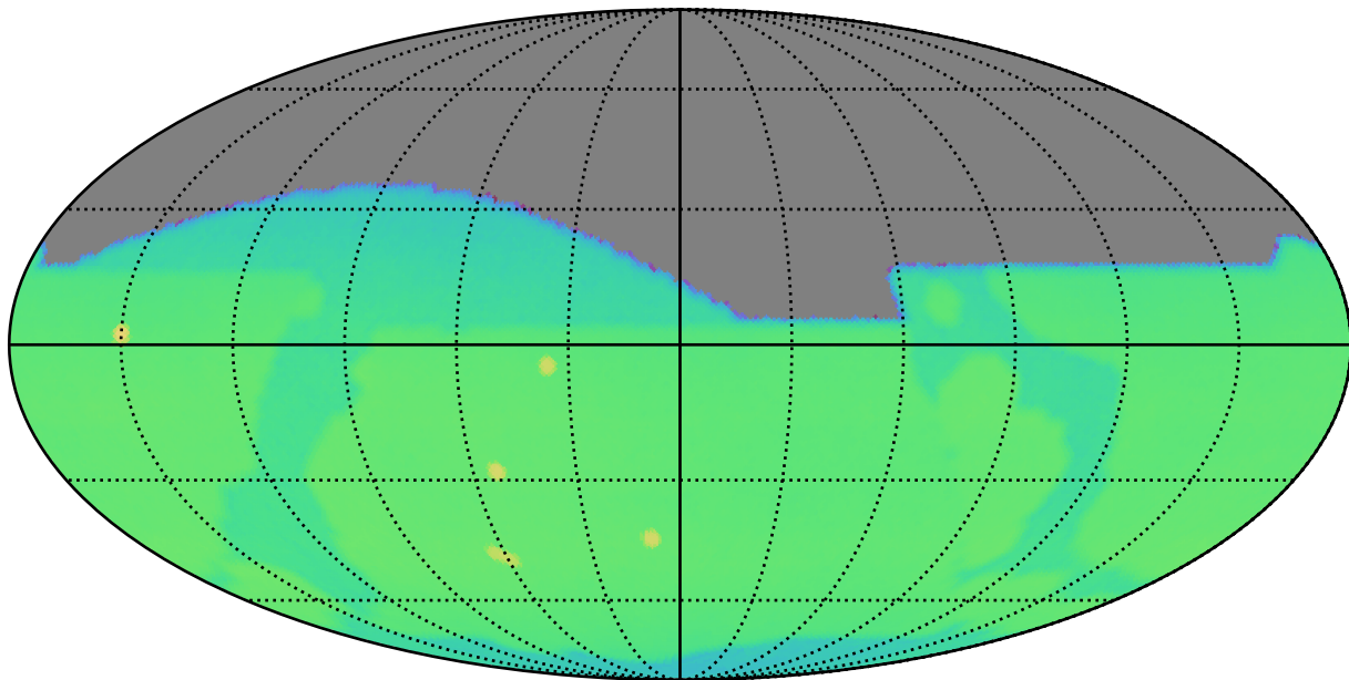
weather_cloudso6v3.4_10yrs : CoaddM5
