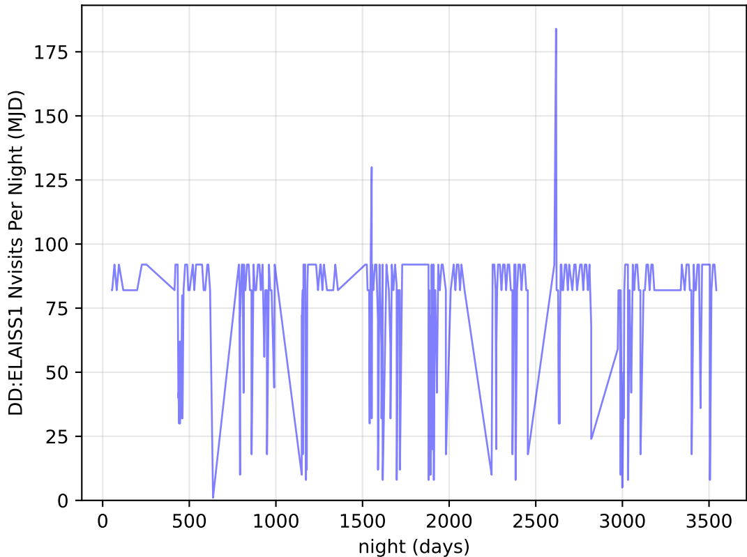
weather_cloudso6v3.4_10yrs all bands: DD:ELAISS1 Nvisits Per Night
