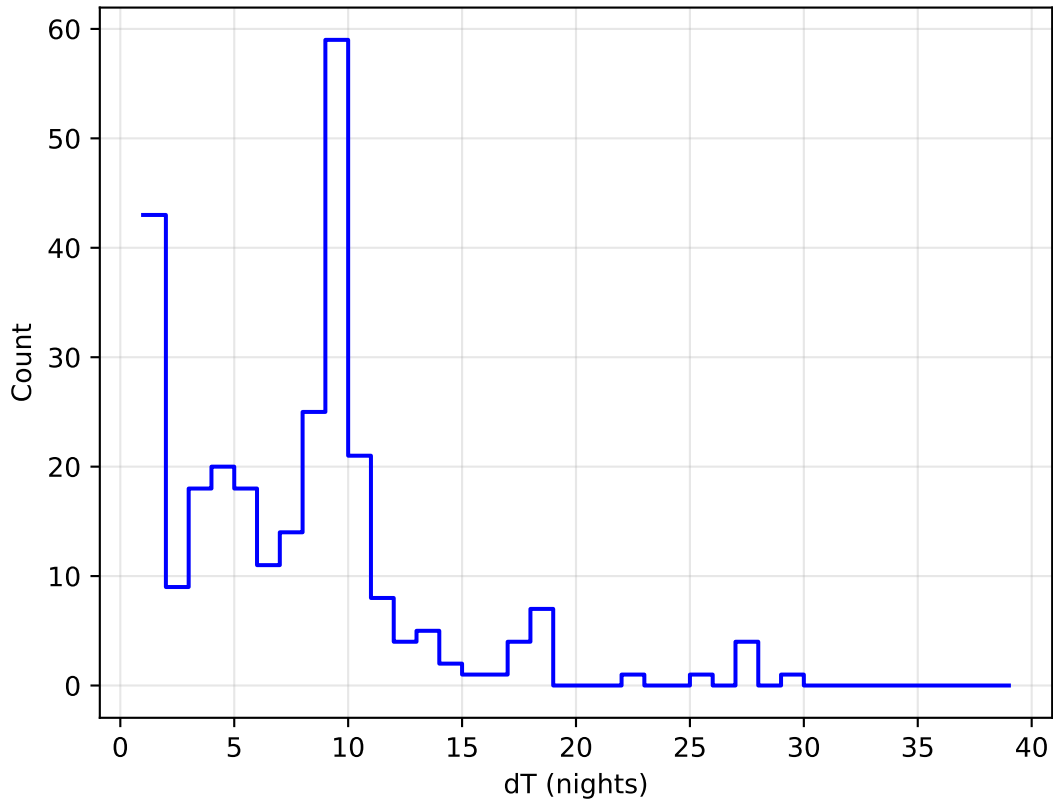
weather_cloudso6v3.4_10yrs all bands: DD:ELAISS1 Delta Nights Histogram
