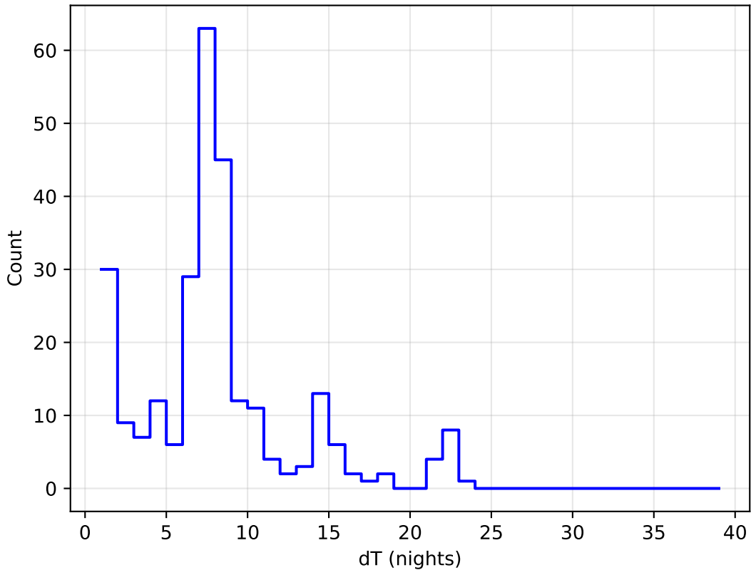
weather_cloudso6v3.4_10yrs all bands: DD:EDFS Delta Nights Histogram
