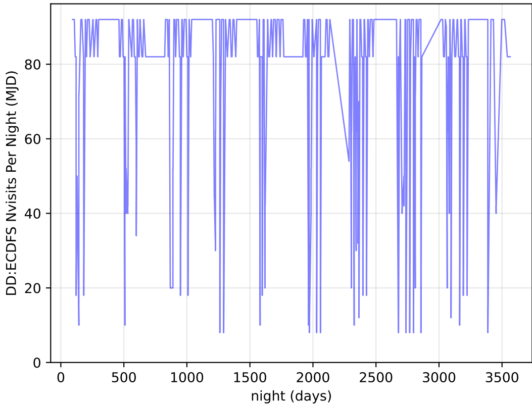
weather_cloudso6v3.4_10yrs all bands: DD:ECDFS Nvisits Per Night
