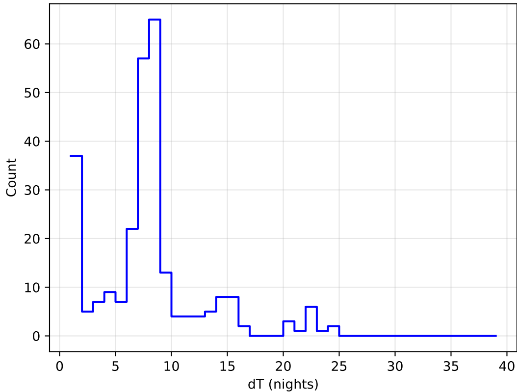
weather_cloudso6v3.4_10yrs all bands: DD:ECDFS Delta Nights Histogram
