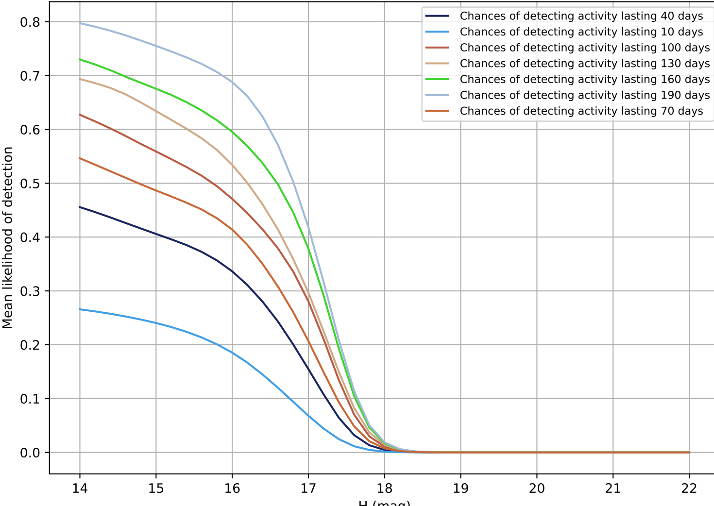
weather_cloudso4v3.4_10yrs Trojan
