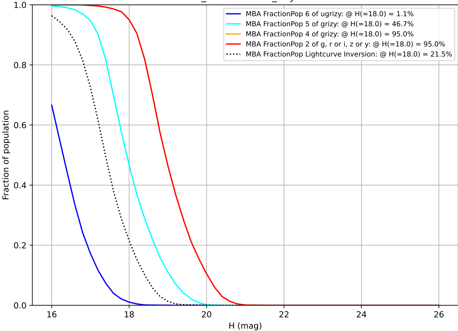
weather_cloudso4v3.4_10yrs MBA
