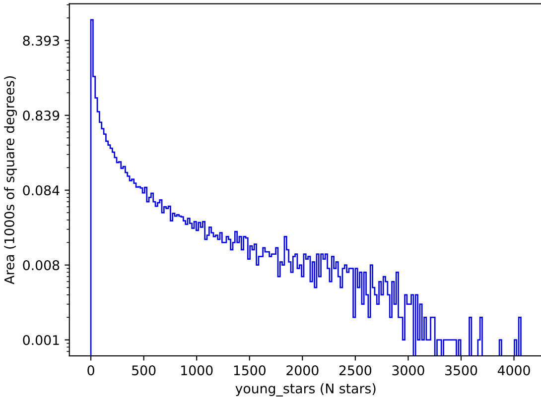
weather_cloudso4v3.4_10yrs : young_stars
