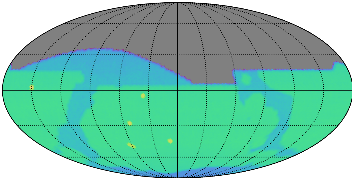
weather_cloudso4v3.4_10yrs i: SurfaceBrightLimit
