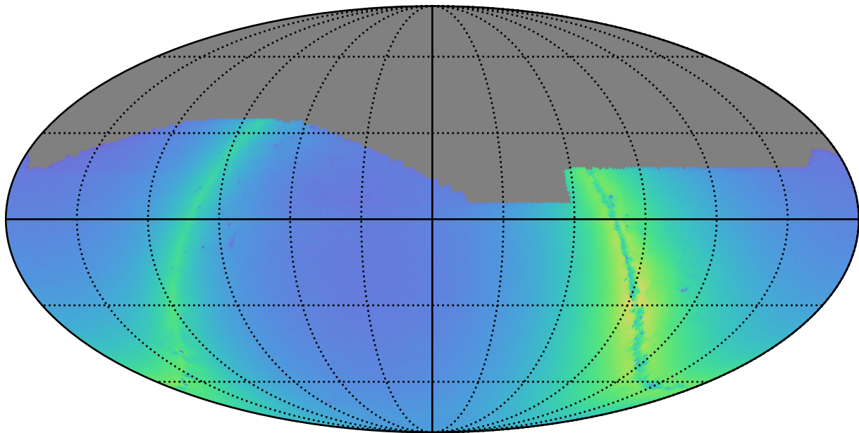
weather_cloudso4v3.4_10yrs z: Nstars_no_crowding
