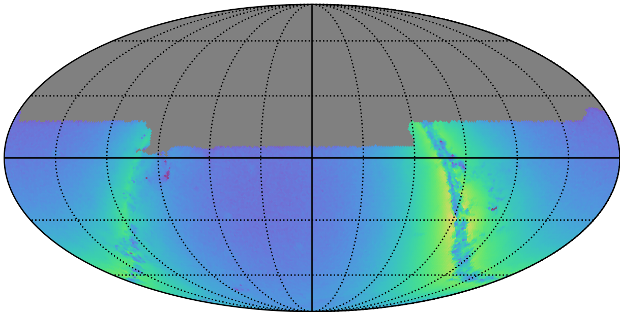
weather_cloudso4v3.4_10yrs u: Nstars_no_crowding
