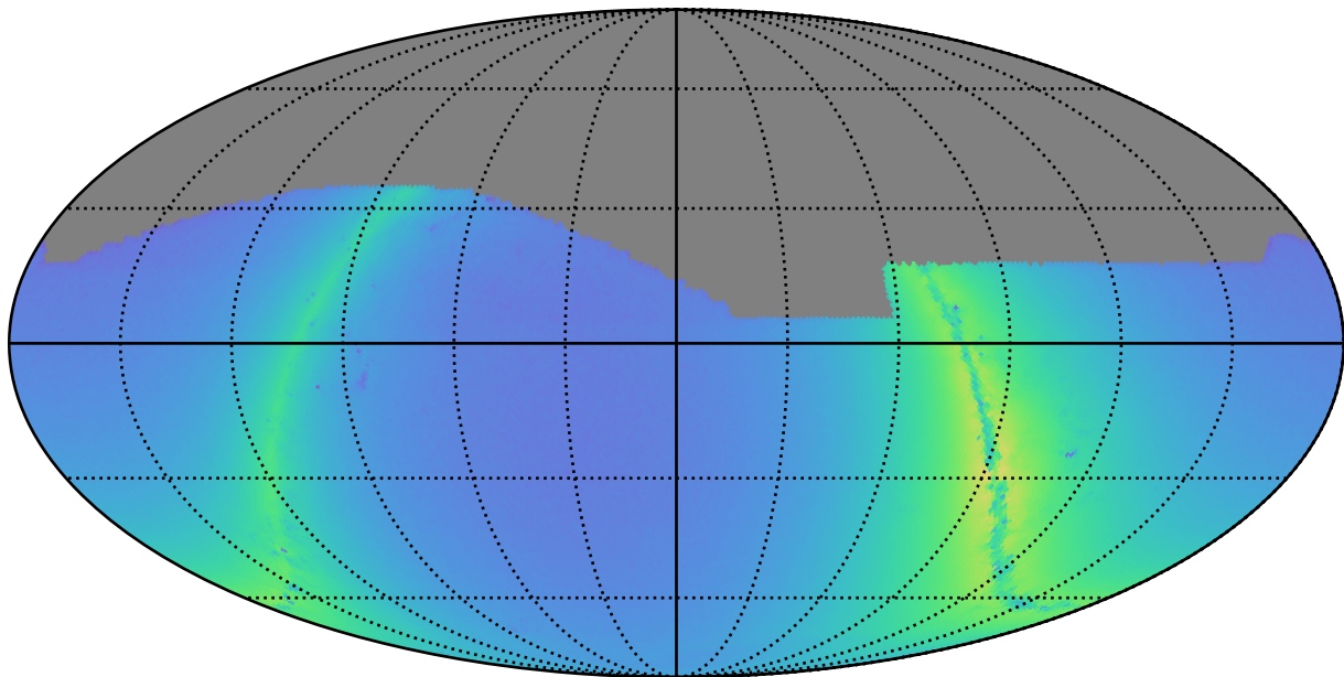
weather_cloudso4v3.4_10yrs i: Nstars_no_crowding
