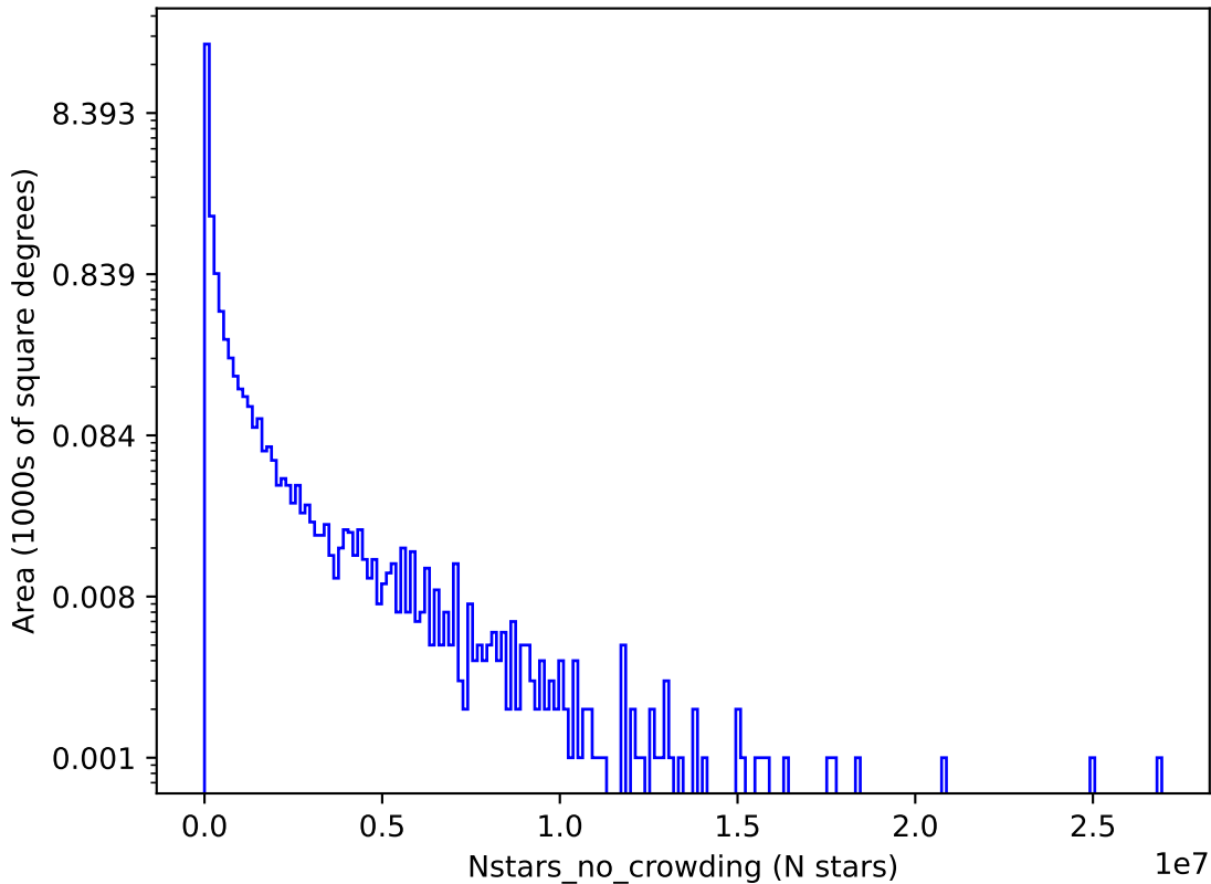
weather_cloudso4v3.4_10yrs i: Nstars_no_crowding
